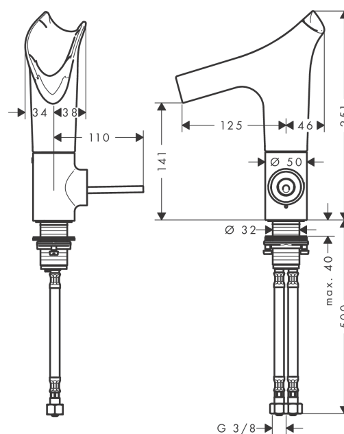
Plan géométral
